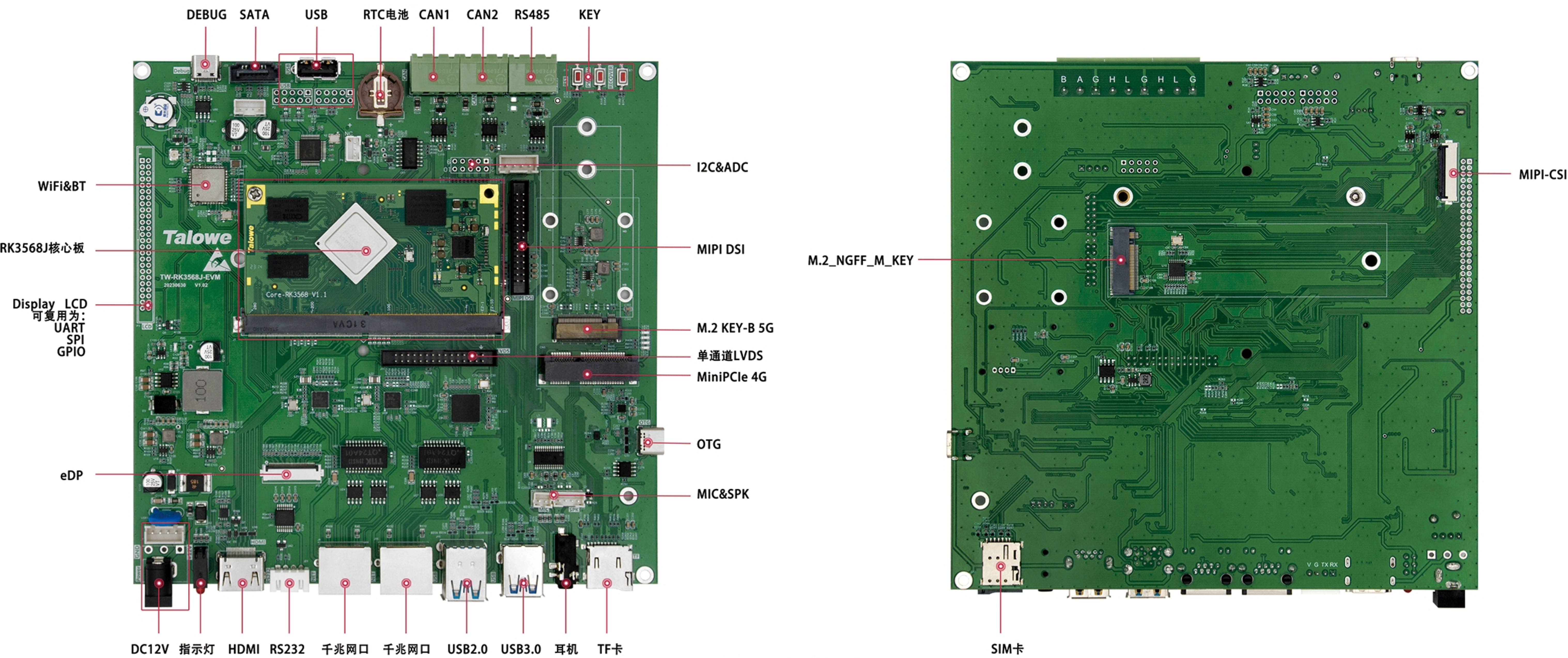
ITX-RK3568评估底板
