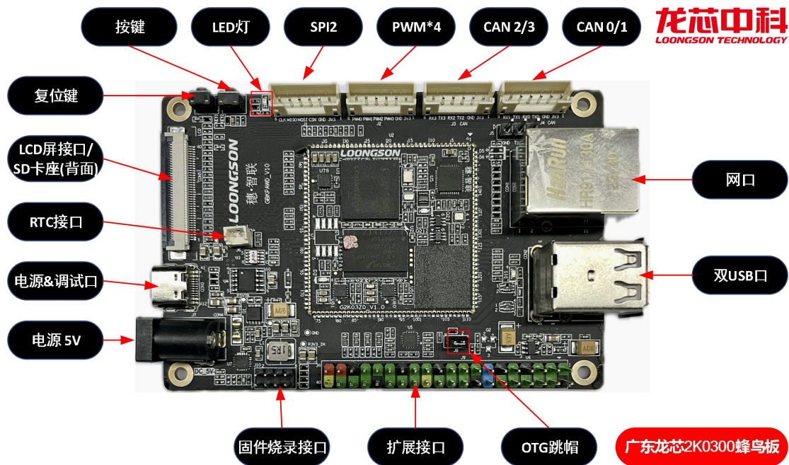
广东龙芯 2K0300 蜂鸟板接口图
