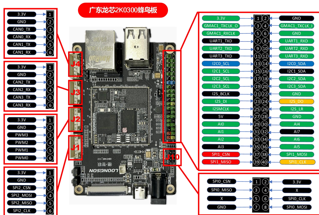
广东龙芯 2K0300 蜂鸟板扩展接口图
